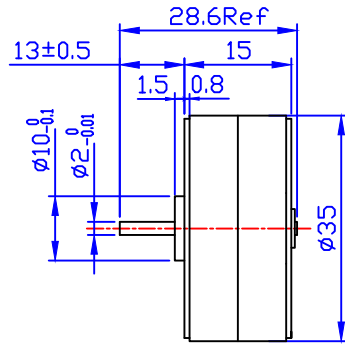
外形图 DIMENSIONS (unit=mm)
