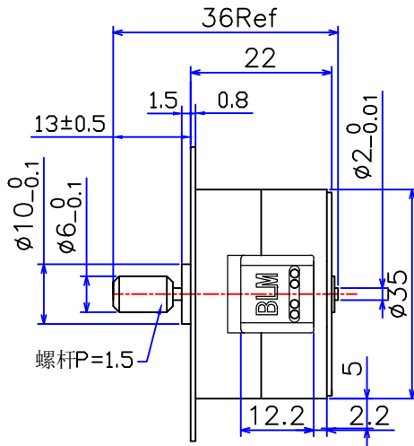
□ 外形图 DIMENSIONS (unit=mm)
